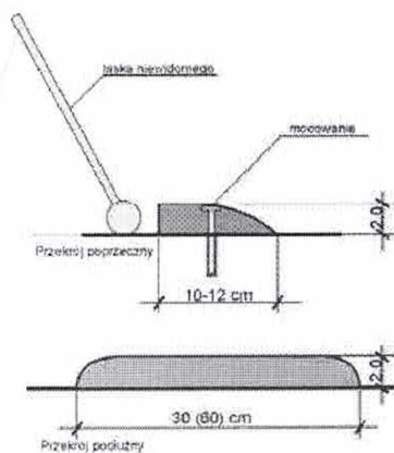
Ryc. A.4. Projekt profilu rozdzielającego ruch rowerowy od pieszego (D3) do zastosowania na istniejących ciągach pieszo-rowerowych (oprac. własne)
