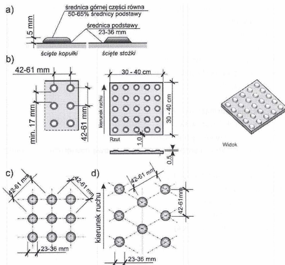
Ryc. A.2. Faktura bezpieczeństwa (typ B) tzw. "ścięte kopytka", "ścięte stożki". (źródło ADAAG)
